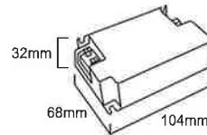
model no. : GFN-TFLTVC18A Drive, INPUT : 100-240V MAX : 18W (350mA)
